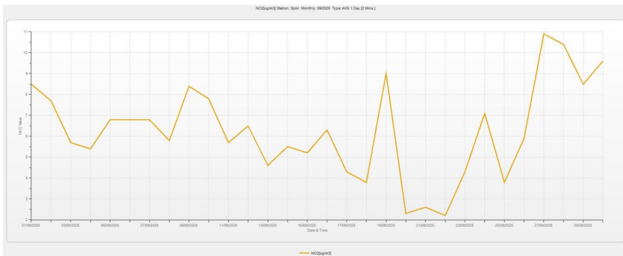
Kuva 4. Typpidioksidin vuorokausipitoisuus syyskuussa 2025.
