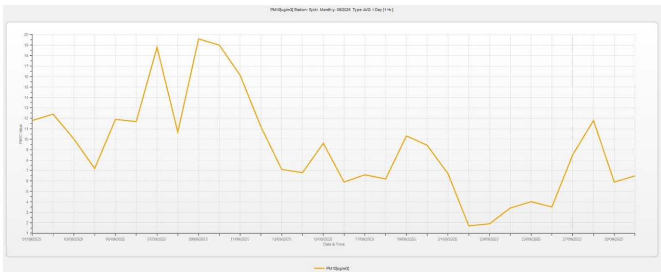
Kuva 2. Hengitettävien hiukkasten vuorokausipitoisuus syyskuussa 2025.
