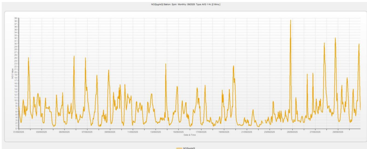
Kuva 3. Typpidioksidin tuntipitoisuus syyskuussa 2025.
