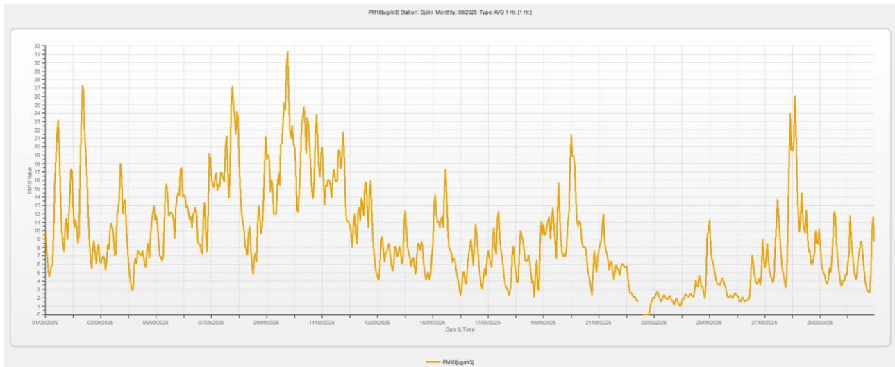
Kuva 1. Hengitettävien hiukkasten tuntipitoisuus syyskuussa 2025.
