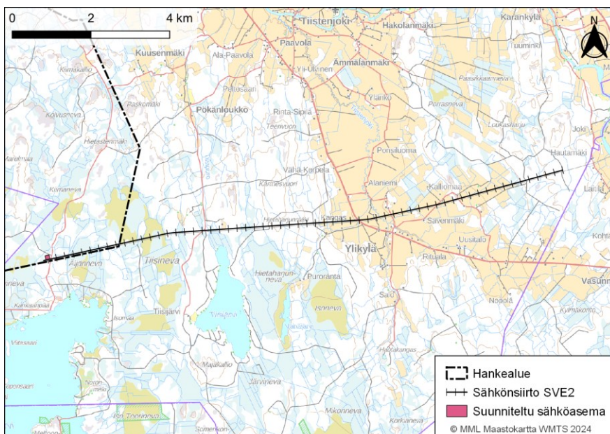
Kuva 4. Lamminnevan sähkönsiirto vaihtoehdoissa SVE 2.
