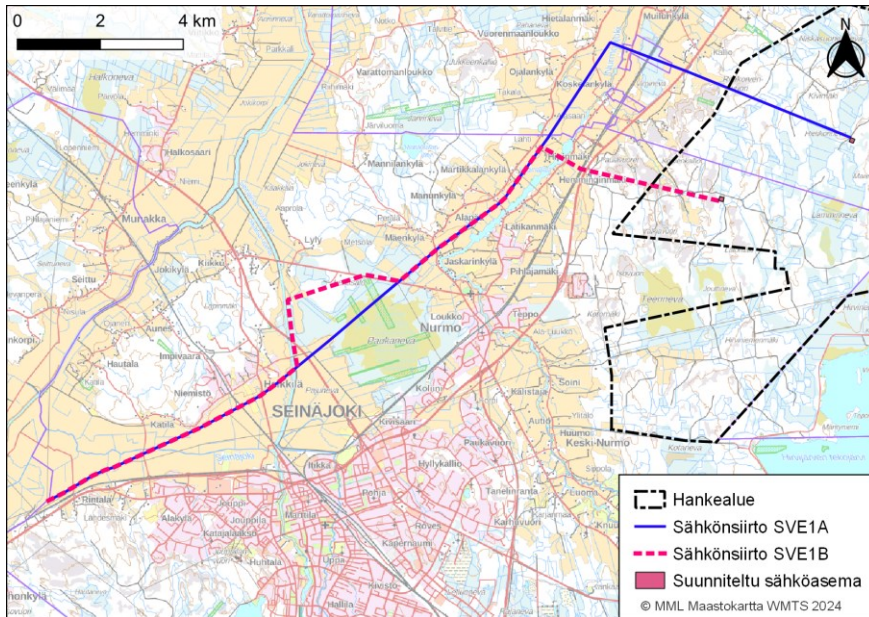
Kuva 3. Lamminnevan sähkönsiirto vaihtoehdoissa SVE 1A ja SVE 1B.
