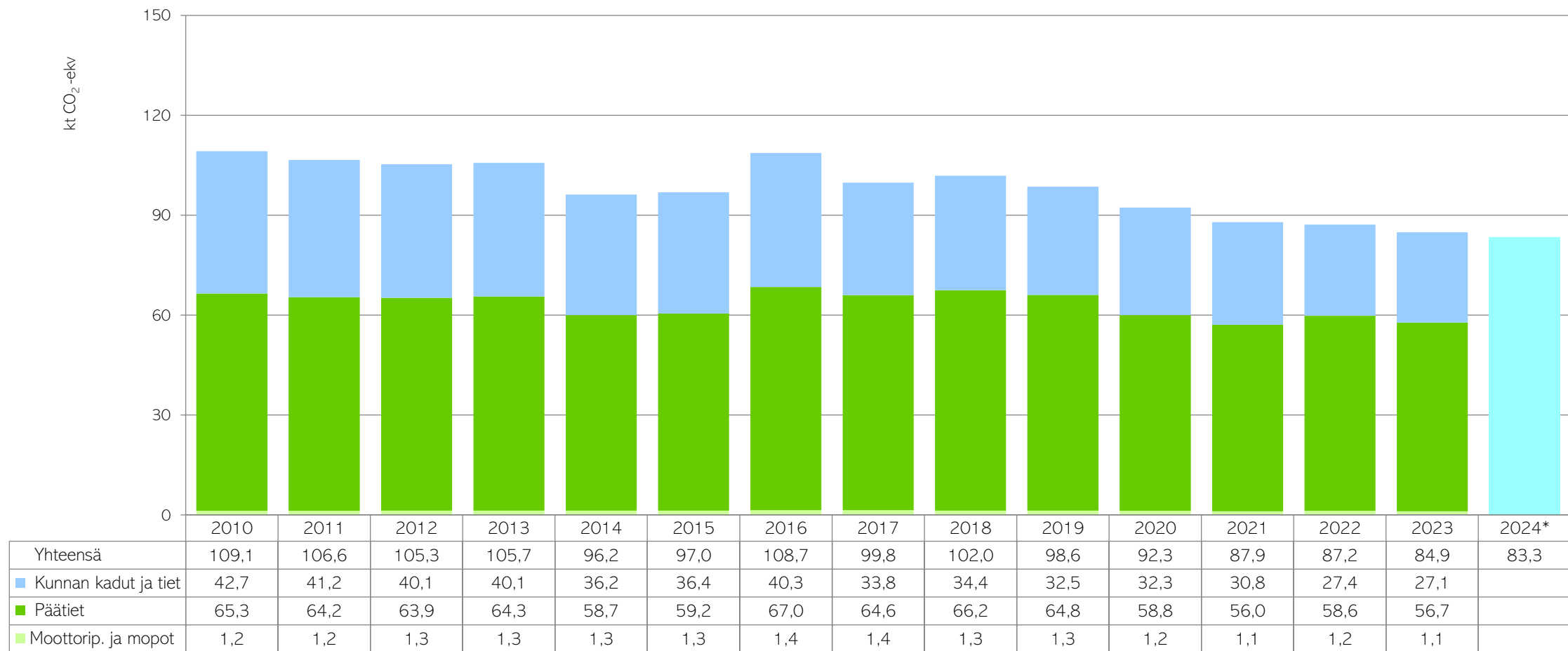
Kuva 7. Tieliikenteen päästöt Seinäjoella vuosina 2010–2024. Vuoden 2024 tieto on ennakkotieto. (CO 2 -raportti, 2025)
