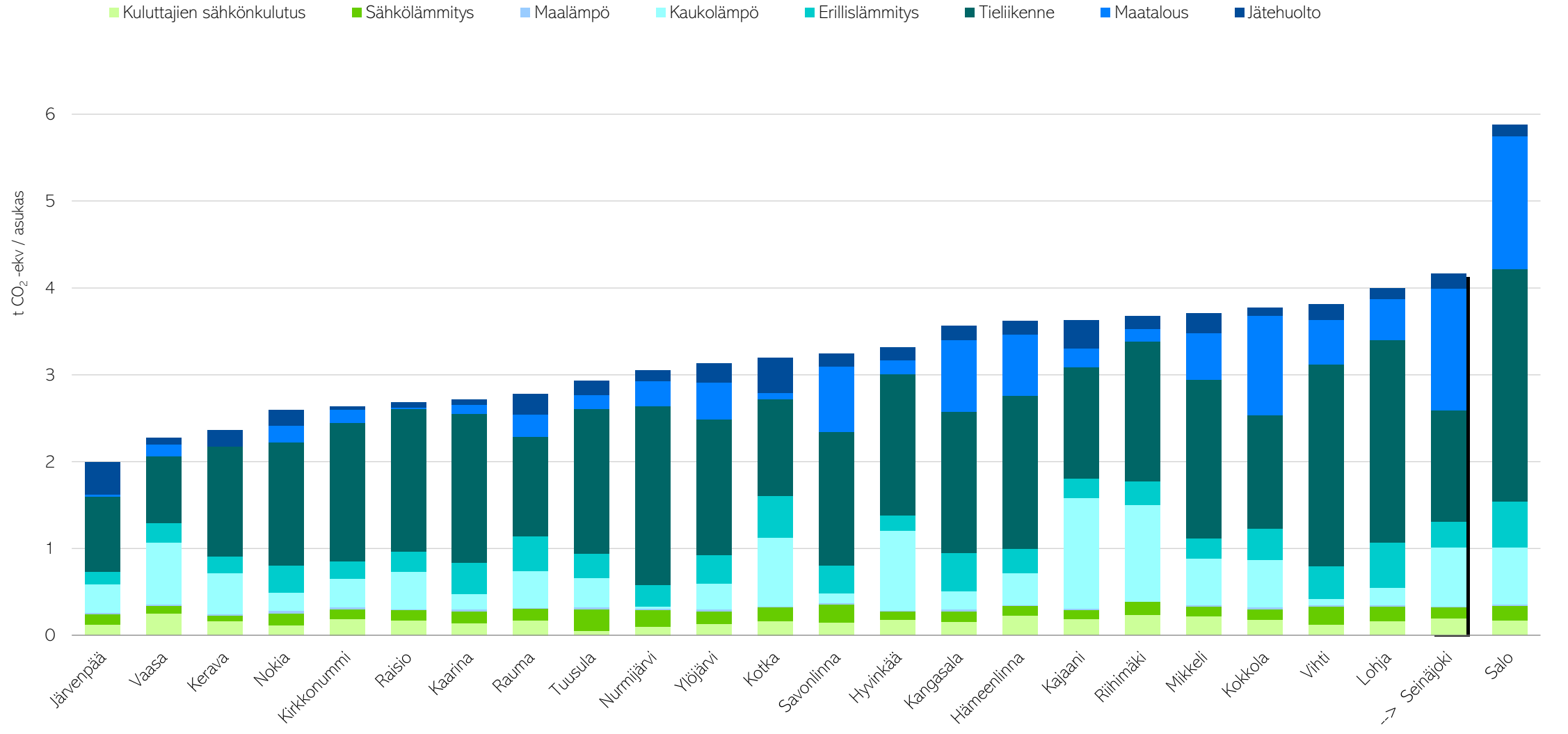
Kuva 12. CO2-raportissa mukana olevien 25 000–70 000 asukkaan kuntien asukaskohtaiset päästöt (t CO 2 -ekv/asukas) vuonna 2023 ilman teollisuutta. (CO 2 -raportti, 2025)
