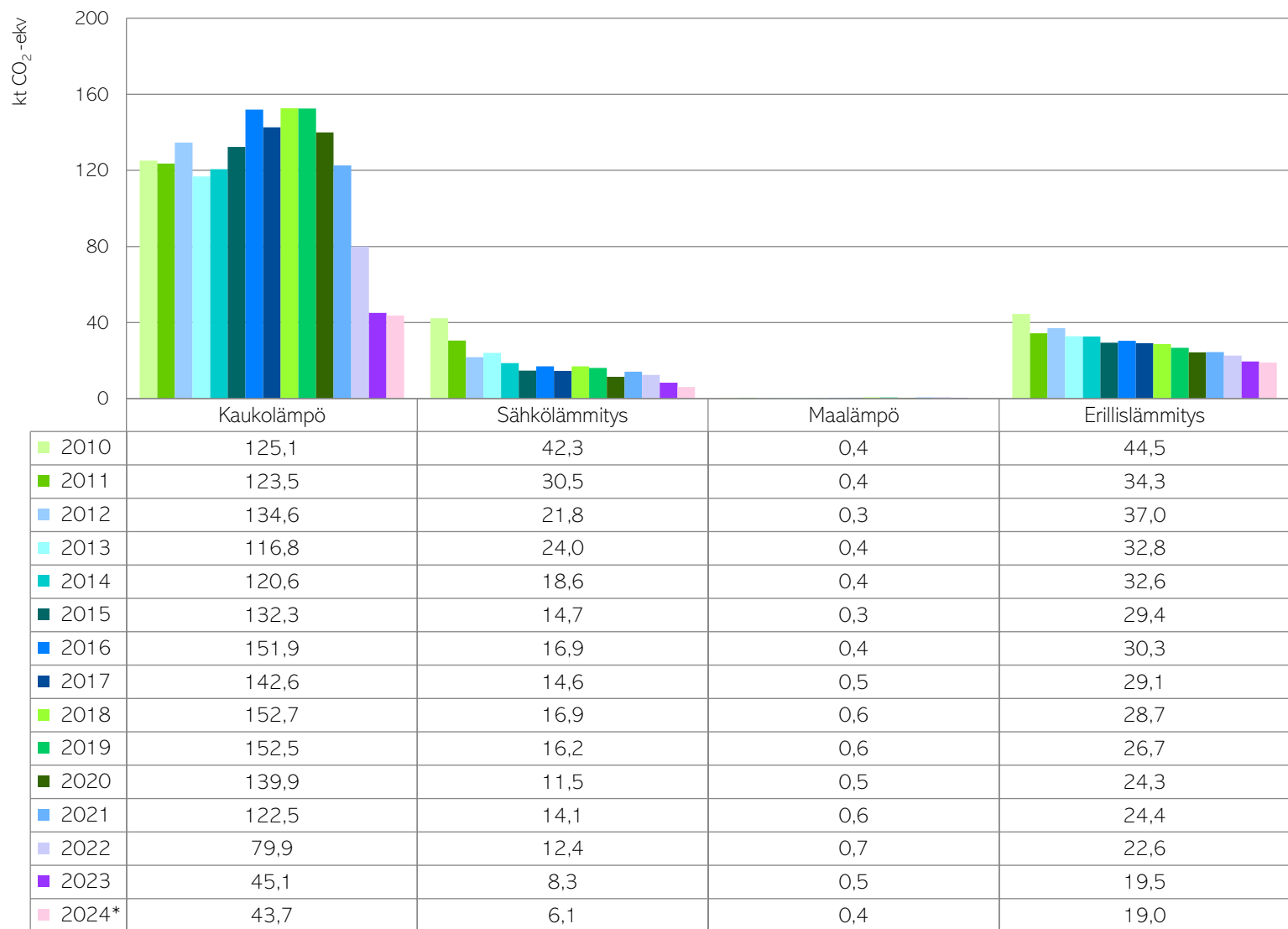
Kuva 6. Rakennusten lämmityksen päästöjen kehitys Seinäjoella vuosina 2010–2024. Vuoden 2024 tieto on ennakkotieto. (CO 2 -raportti, 2025)
