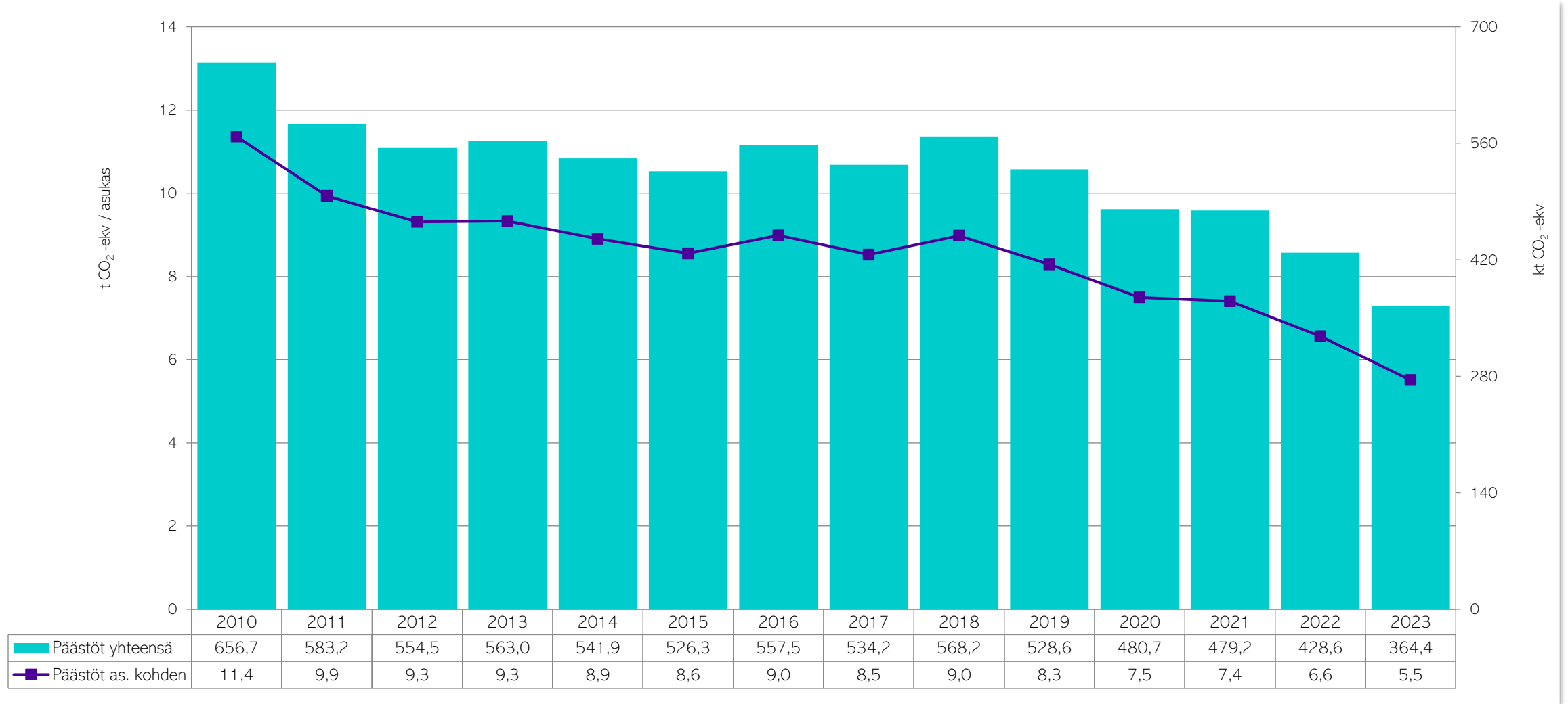
Kuva 4. Päästöt yhteensä ja asukasta kohden Seinäjoella vuosina 2010–2023, kun teollisuuden päästöt ovat mukana tarkastelussa. (CO 2 -raportti, 2025)
