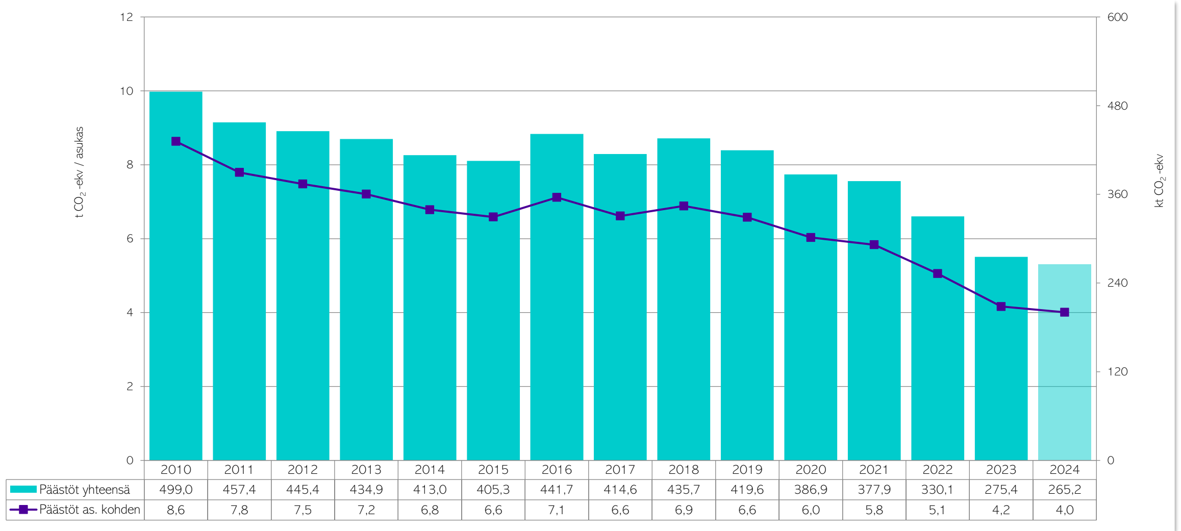
Kuva 3. Päästöt yhteensä ja asukasta kohden Seinäjoella vuosina 2010–2024 ilman teollisuutta. Vuoden 2024 tieto on ennakkotieto. (CO 2 -raportti, 2025)
