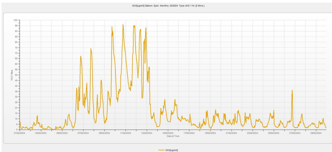
Kuva 3. Typpidioksidin tuntipitoisuus helmikuussa 2024.
