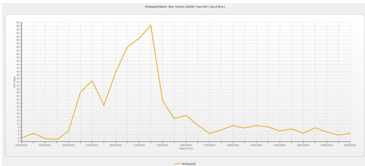
Kuva 4. Typpidioksidin vuorokausipitoisuus helmikuussa 2024.
