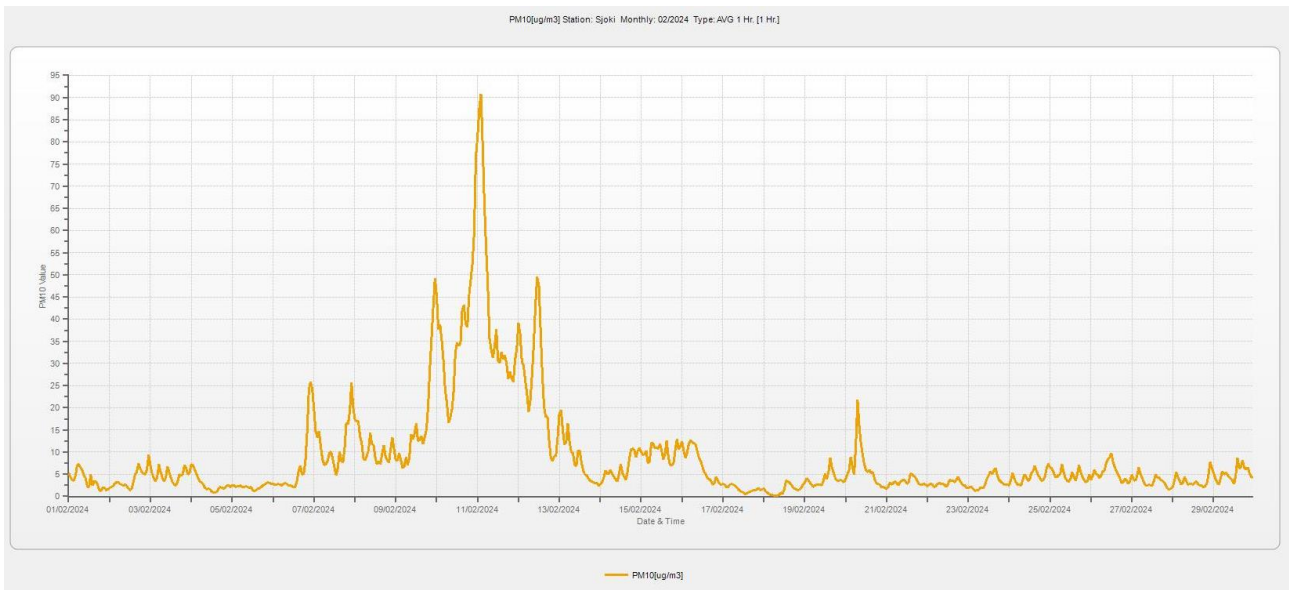
Kuva 1. Hengitettävien hiukkasten tuntipitoisuus helmikuussa 2024.
