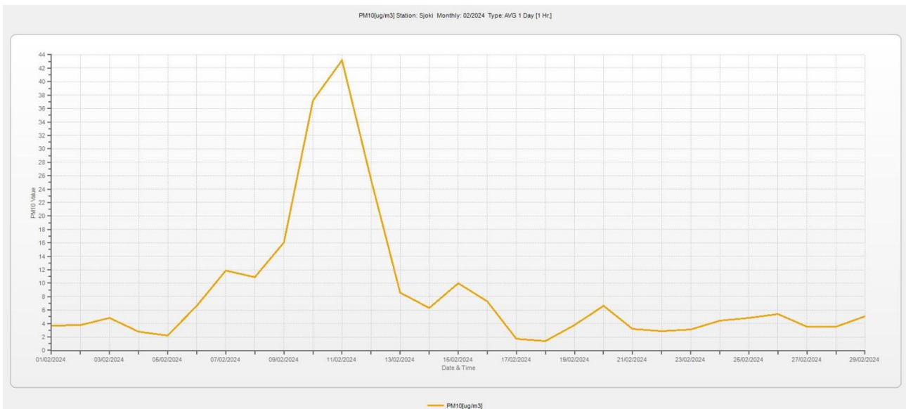
Kuva 2. Hengitettävien hiukkasten vuorokausipitoisuus helmikuussa 2024.
