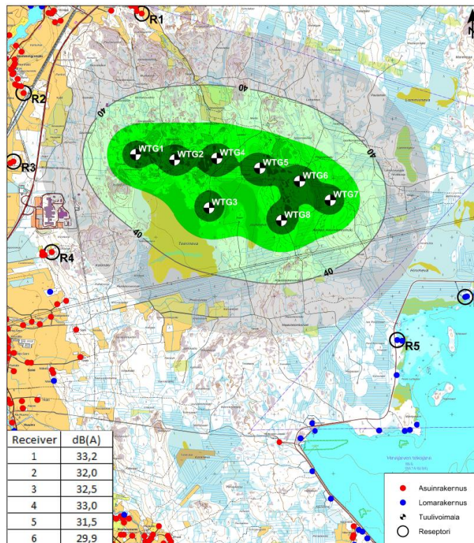
Kuva 1. Reseptoripisteiden R1-R6 sijainnit. Kuvassa VE1 mukainen voimalasijoittelu.
