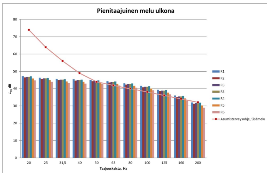
Kuva 5. VE2 pienitaajuisen ulkomelun laskentatulokset reseptoripisteissä
