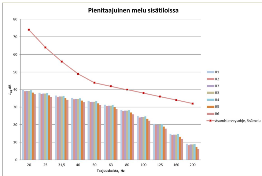
Kuva 4. VE2 pienitaajuisen sisämelun laskentatulokset reseptoripisteissä
