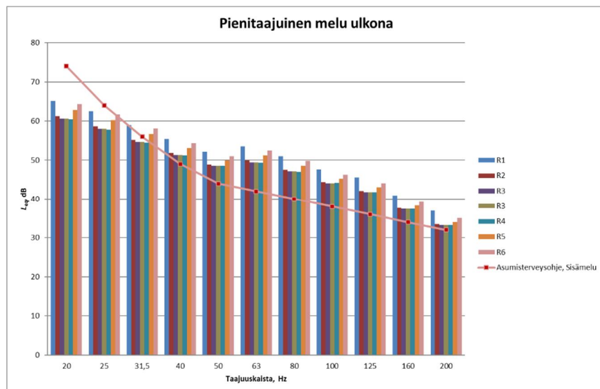
Kuva 13. Yhteismallinnuksen VE2+Fortum VE2 pienitaajuisen ulkomelun laskentatulokset reseptoripisteissä
