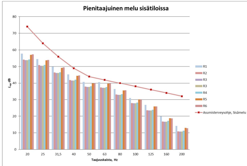
Kuva 8. Yhteismallinnuksen VE2+Fortum VE1 pienitaajuisen sisämelun laskentatulokset reseptoripisteissä
