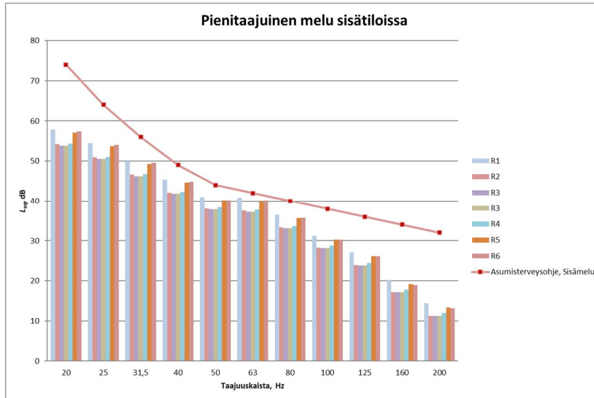
Kuva 6. Yhteismallinnuksen VE1+Fortum VE1 pienitaajuisten sisämelun laskentatulokset reseptoripisteissä
