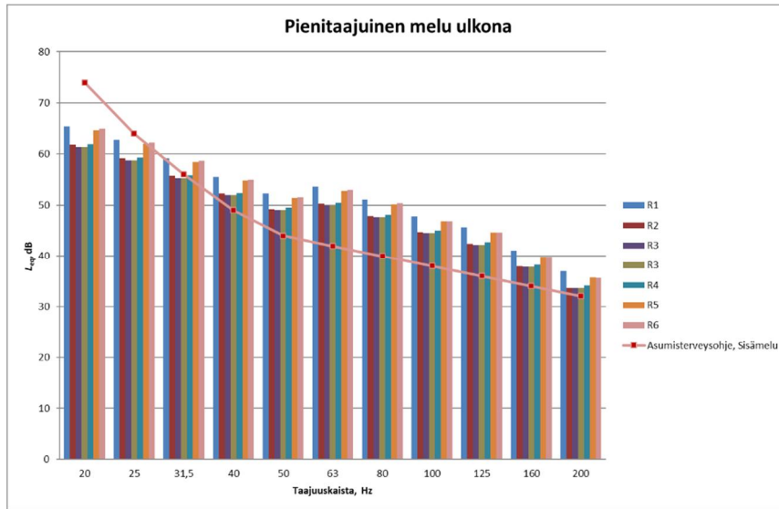
Kuva 9. Yhteismallinnuksen VE2+Fortum VE1 pienitaajuisen ulkomelun laskentatulokset reseptoripisteissä
