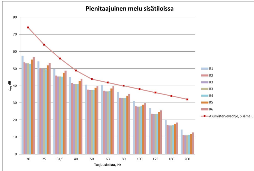
Kuva 10. Yhteismallinnuksen VE1 + Fortum VE2 pienitaajuisen sisämelun laskentatulokset reseptoripisteissä
