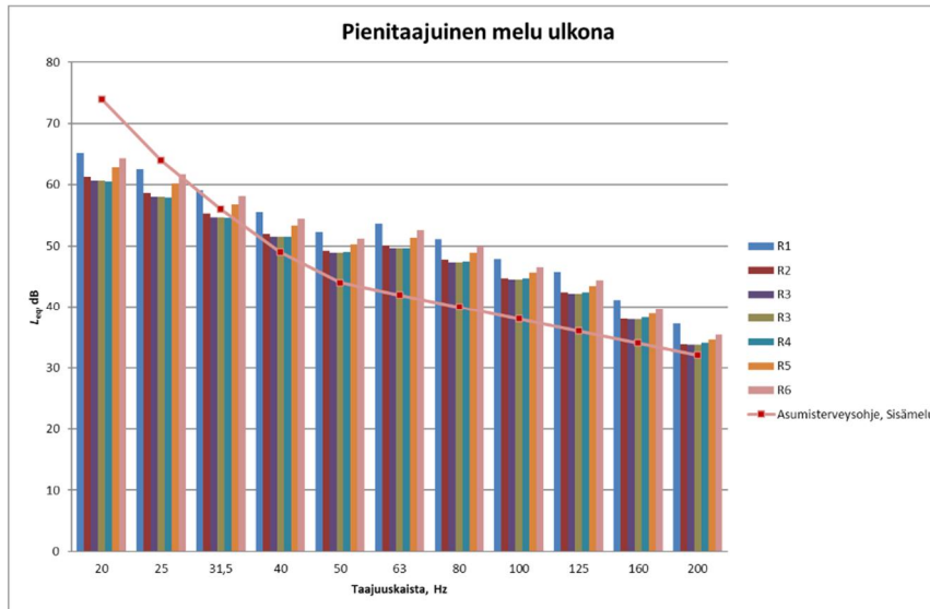
Kuva 11. Yhteismallinnuksen VE1 + Fortum VE2 pienitaajuisen ulkomelun laskentatulokset reseptoripisteissä
