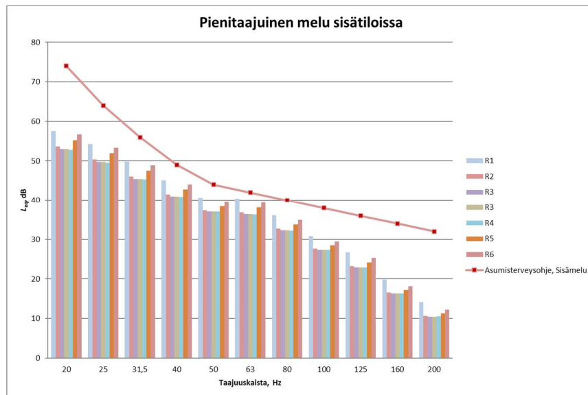
Kuva 12. Yhteismallinnuksen VE2+Fortum VE2 pienitaajuisen sisämelun laskentatulokset reseptoripisteissä
