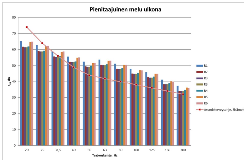
Kuva 7. Yhteismallinnuksen VE1+Fortum VE1 pienitaajuisten ulkomelun laskentatulokset reseptoripisteissä
