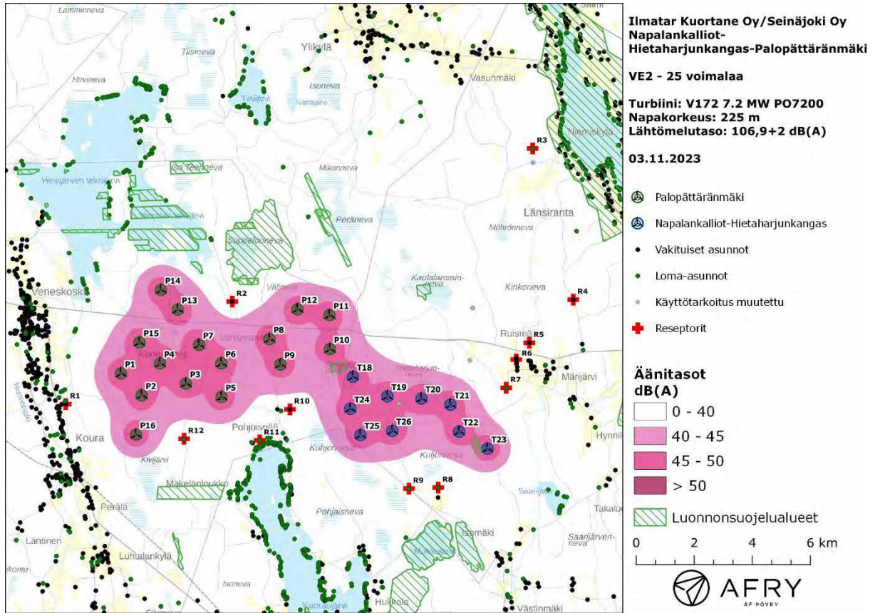
Kuva 6: Keskiäänitasot LAeq tuulivoimapauston hankealueella toteutusvaihtoehdolla VE2.
