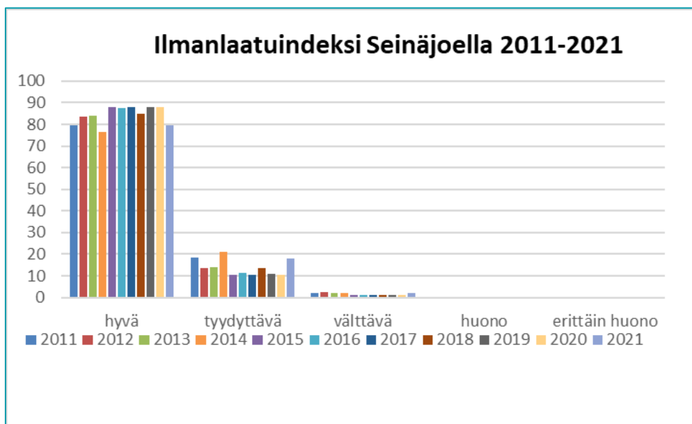
Kuva 17. Ilmanlaatuindeksi Seinäjoella 2011-2021.
