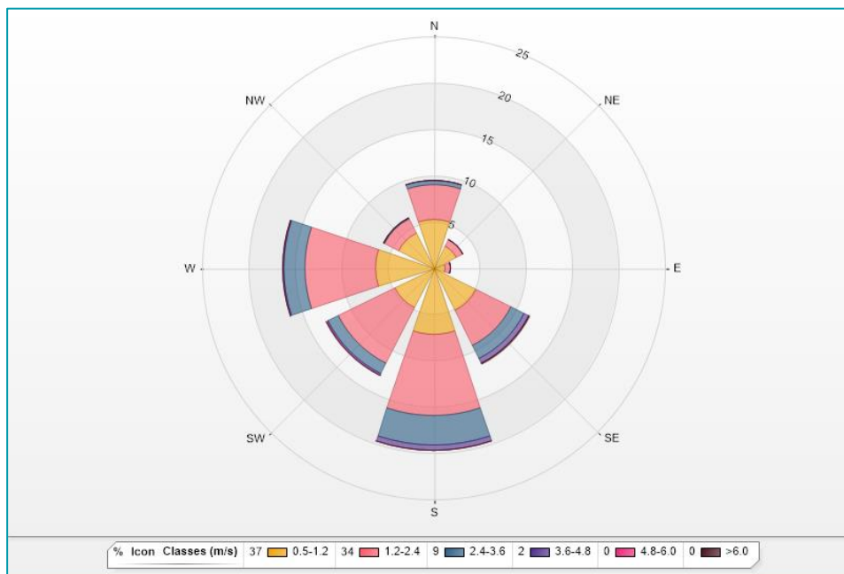
Kuva 20. Tuulen suunta ja nopeus Vapaudentien mittausasemalla 2021.
