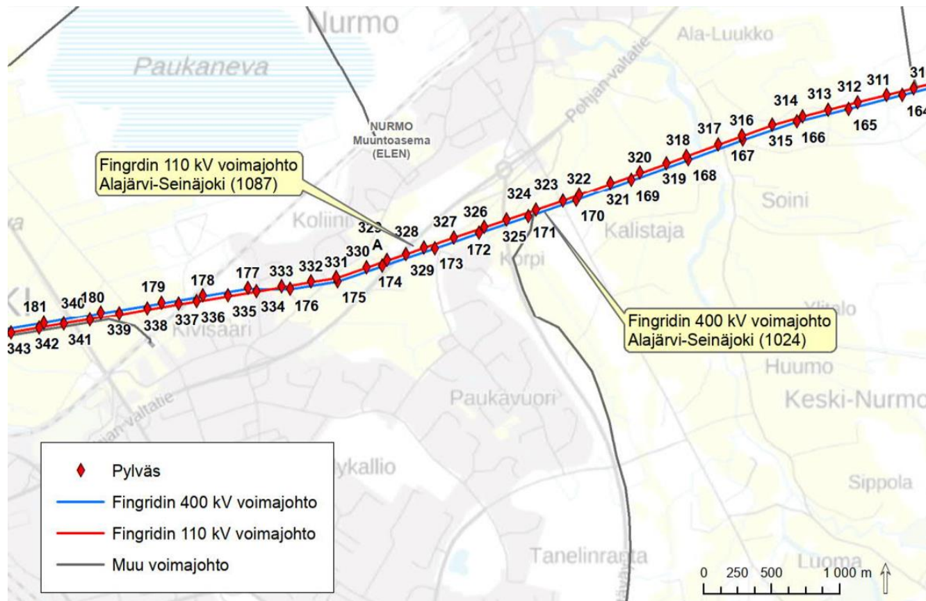
Kuva 1. Voimajohtojen sijainti:
