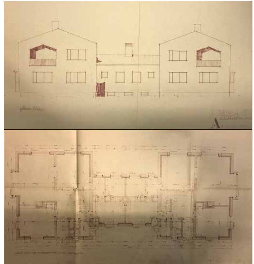
Rakennuksen eteläsivu ja ensimmäisen kerroksen pohjapiirros arkkitehtitoimisto Cederc-reutz & Railon vuonna 1949 laatimissa alkuperäispiirustuksissa. (Rakennuspiirros Seinäjoen kaupungin rakennusvalvonnan arkisto.)
