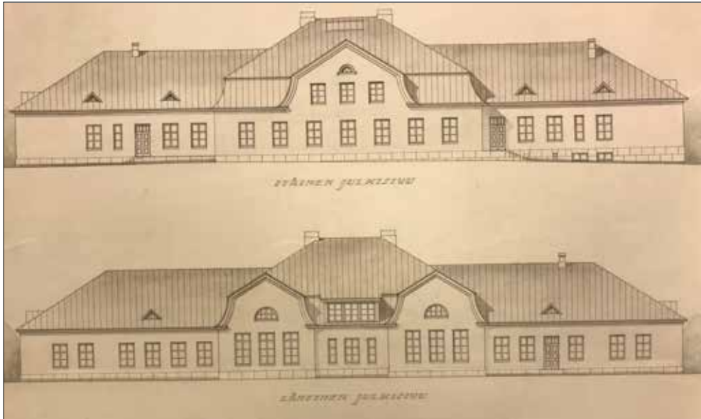
Rakennuksen ulkoasu muuttui merkittävästi vuosina 1955-56 suunniteltujen muutosten seurauksena. Kuvassa julkisivu länteen. Suunnittelijana toimi arkkitehtitoimisto Cedercreutz & Railo. (Rakennuspiirros Etelä-Pohjanmaan sairaanhoitopiirin arkisto).
