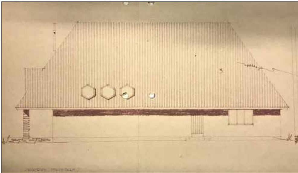
Julksivu pohjoiseen vuoden 1949 rakennuspiirustuksissa. Suunnittelija arkkitehtitoimisto Cedecreutz & Railo. (Rakennuspiirustus Seinäjoen kaupungin rakennusvalvonnan arkisto.)
