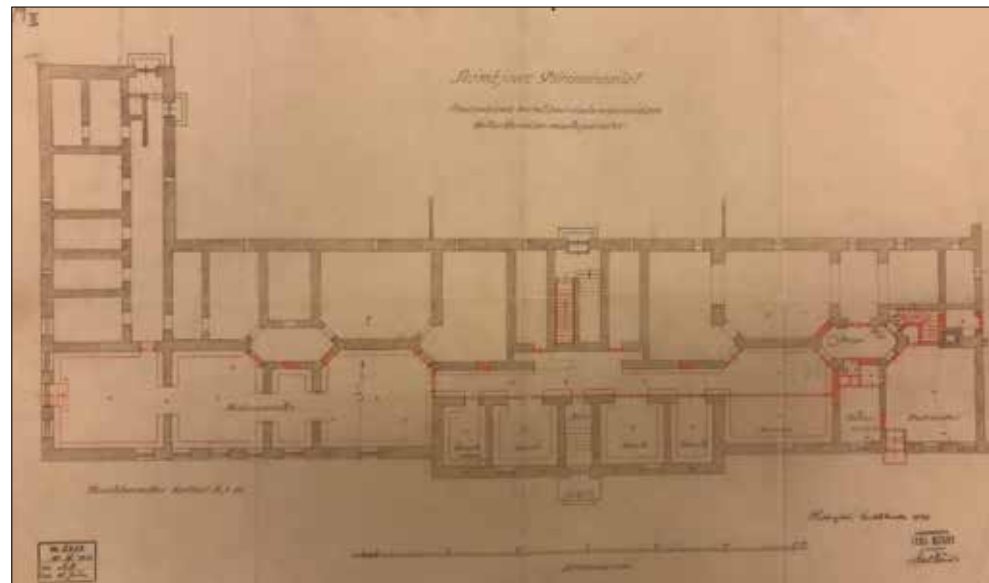
B-rakennuksen kellarikerroksen vuoden 1932 osittainen muutos keskusvarastoksi ja entisen pannuhuoneen muutos postikonttoriksi ja puhelinkeskuksiksi. Suunnittelija arkkitehti Axel Mörne. (Rakennuspiirros Etelä-Pohjanmaan sairaanhoitopiirin arkisto.)
