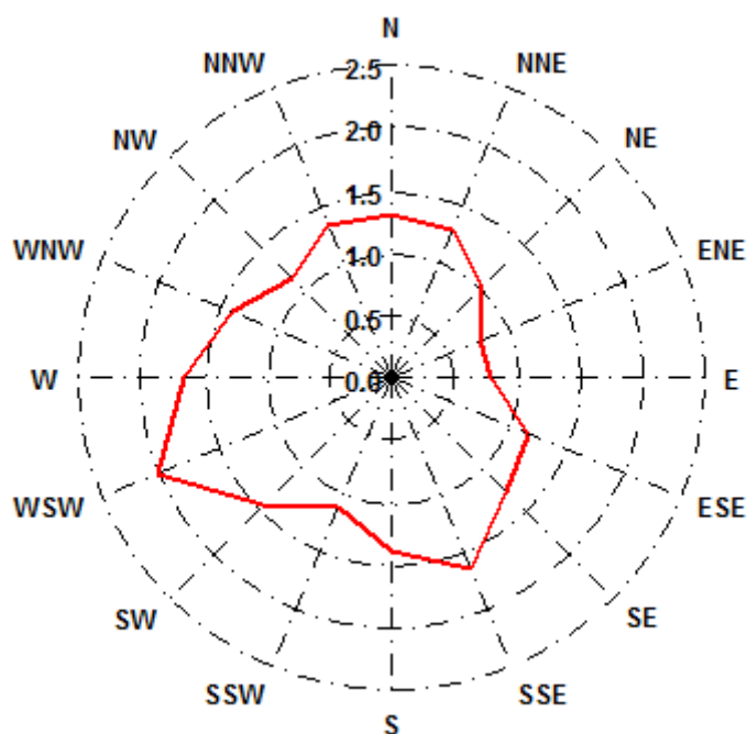
Kuva 17. Tuulen suunta Vapaudentien mittausasemalla 2019
