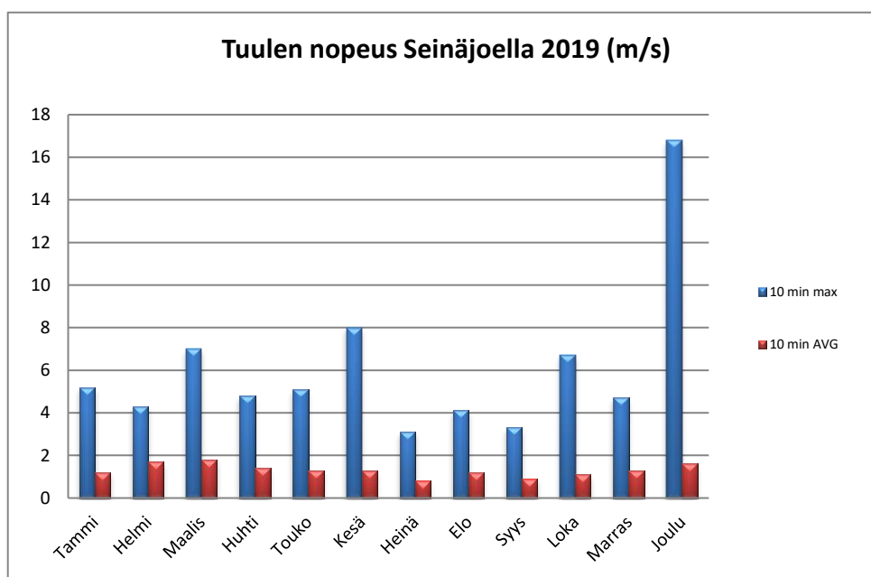
Kuva 18. Tuulen kuukausittaiset maksimiarvot ja keskinopeudet vuonna 2019.
