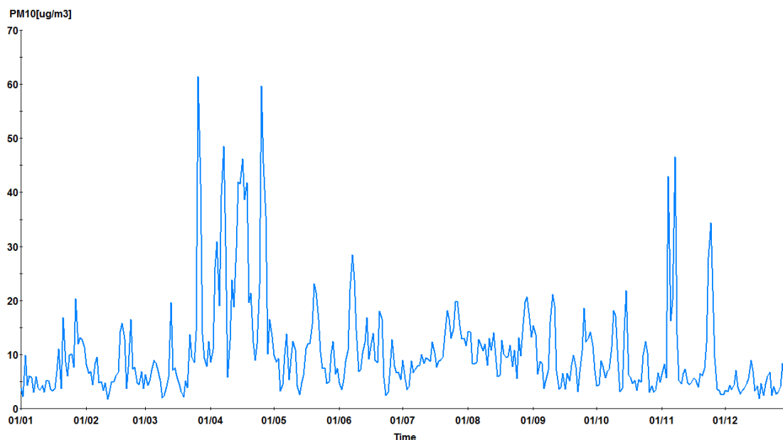
Kuva 12. Hengitettävien hiukkasten (PM 10 ) vuorokausiarvot vuonna 2019.
