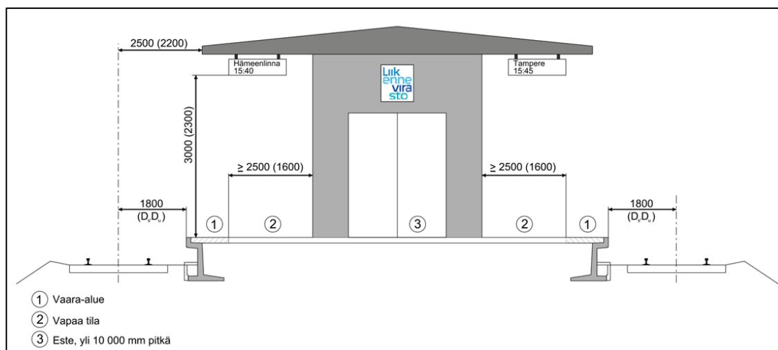
Kuva 11.. RATO 16 Kuva 16.5:9 Välilaiturin vähimmäisleveys, laiturin vapaan tilan korkeus ja laiturikatoksen etäisyys raiteesta, kun laiturilla on yli 10 m pitkä este. Suositeltavat vähimmäismatrat ja suluissa vähimmäisvaatimukset.
