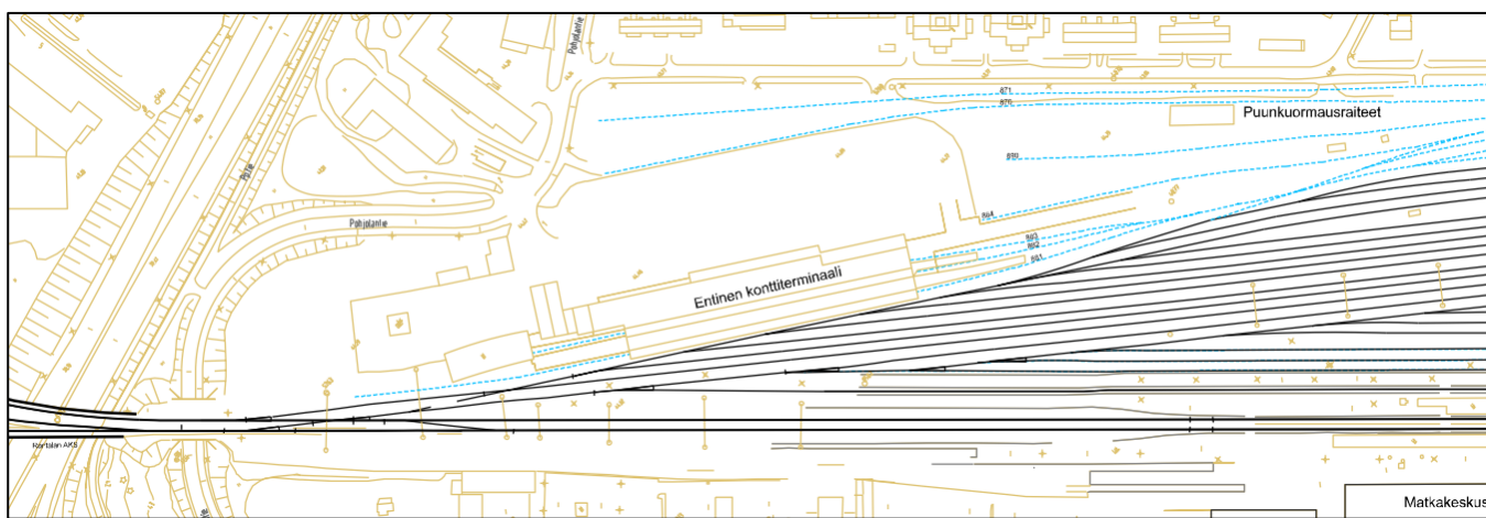
Kuva 8. Karttaote nykyisestä Konttiterminaal- ja puunkuormausalueesta. Sinisellä katkoviivalla on esitetty purettavaksi ehdotetut raiteet.
