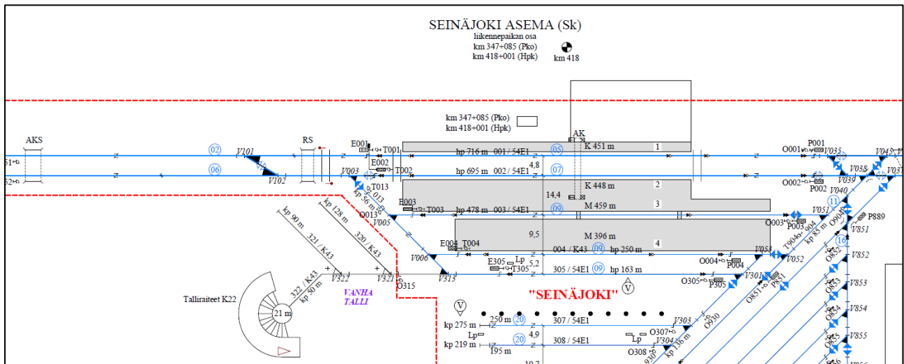
Kuva 10. Karttaote raiteistokaaviosta
