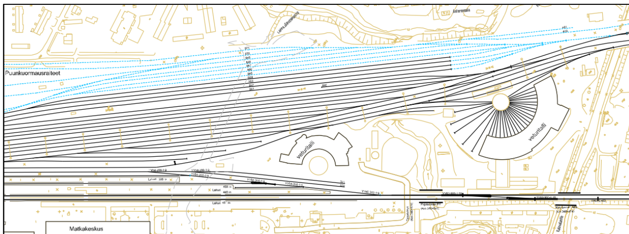
Kuva 9. Karttaote nykyisestä Alaratapihan ja talliraitteiden raiteistosta. Sinisellä katkoviivalla on esitetty purettavaksi ehdotetut raiteet.
