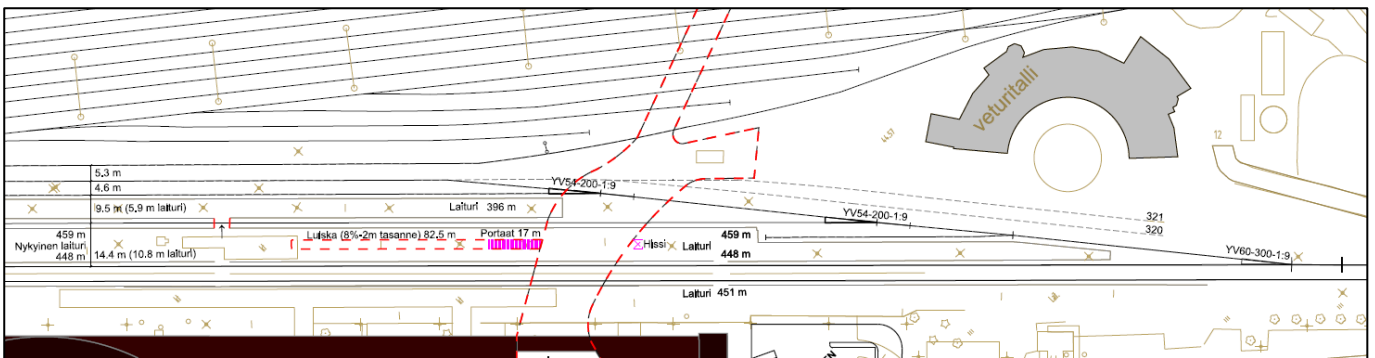
Kuva 13. Karttaote vaihtoehdon 0+ suunnitelmakartasta
