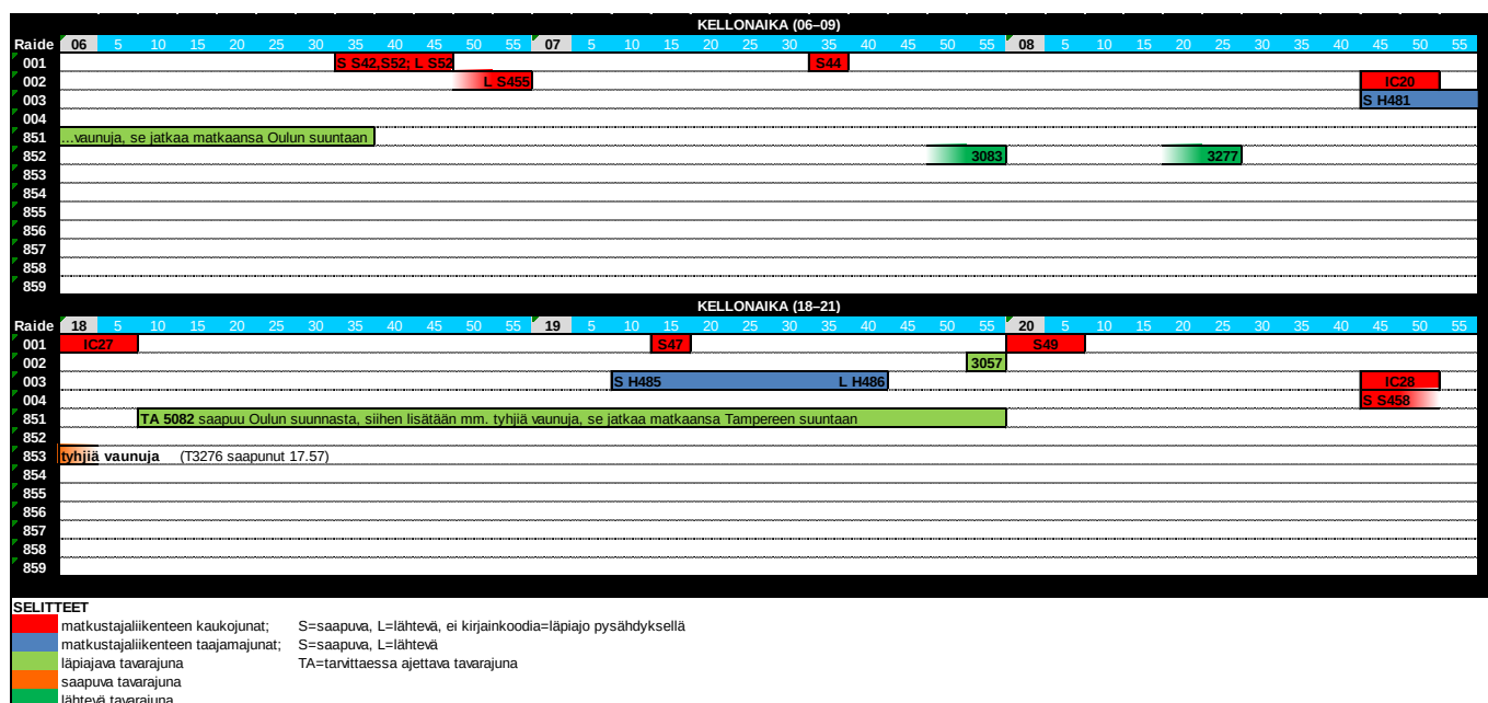
Kuva 7. Seinäjoen ratapihan junien raiteistonkäyttö torstaisin klo 6–9 ja 18–21.
