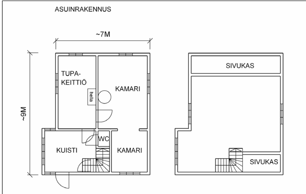
Asuinrakennuksen pohjakaava
