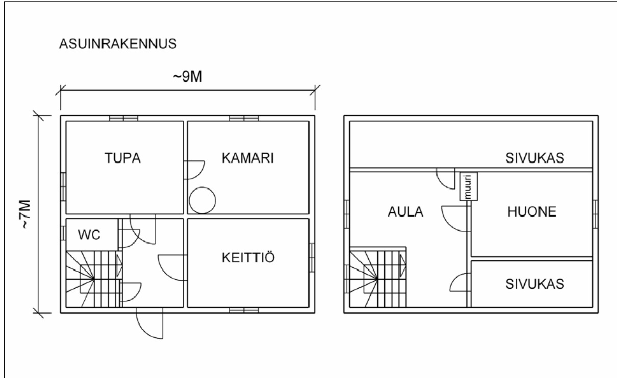
Asuinrakennuksen pohjakaava
