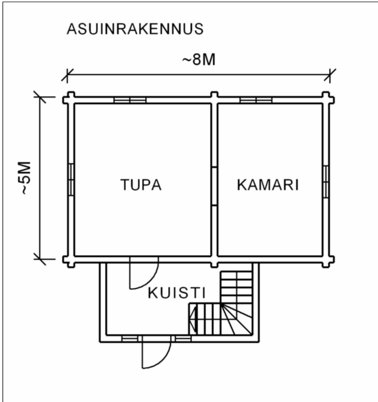
Asuinrakennuksen pohjakaava
