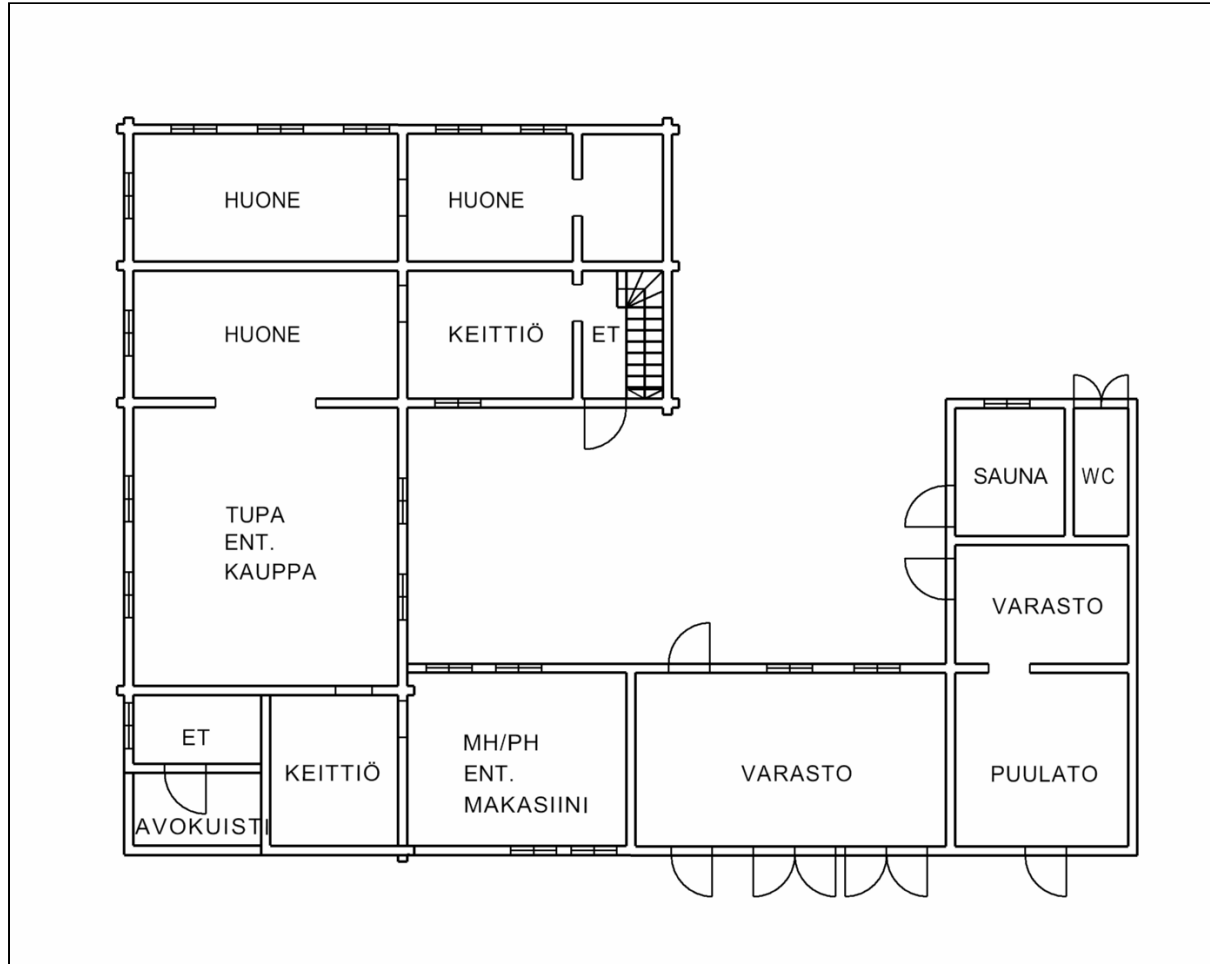
Asuinrakennuksen pohjakaava
