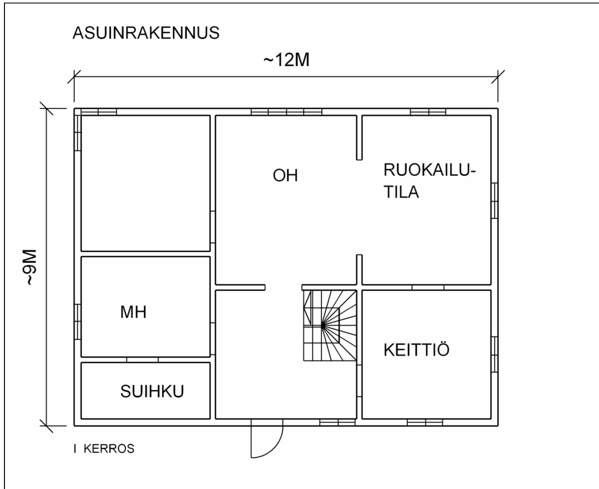
Asuinrakennuksen pohjakaava
