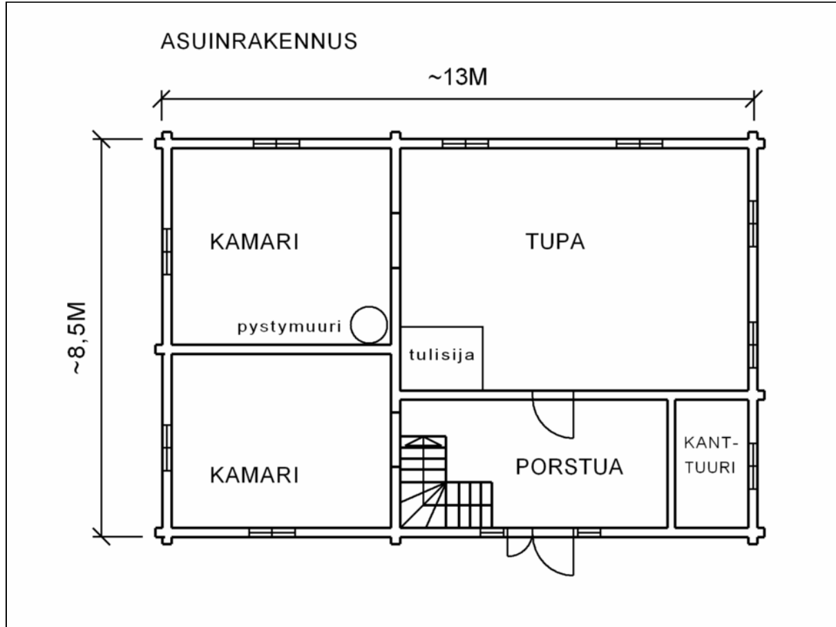
Asuinrakennuksen pohjakaava
