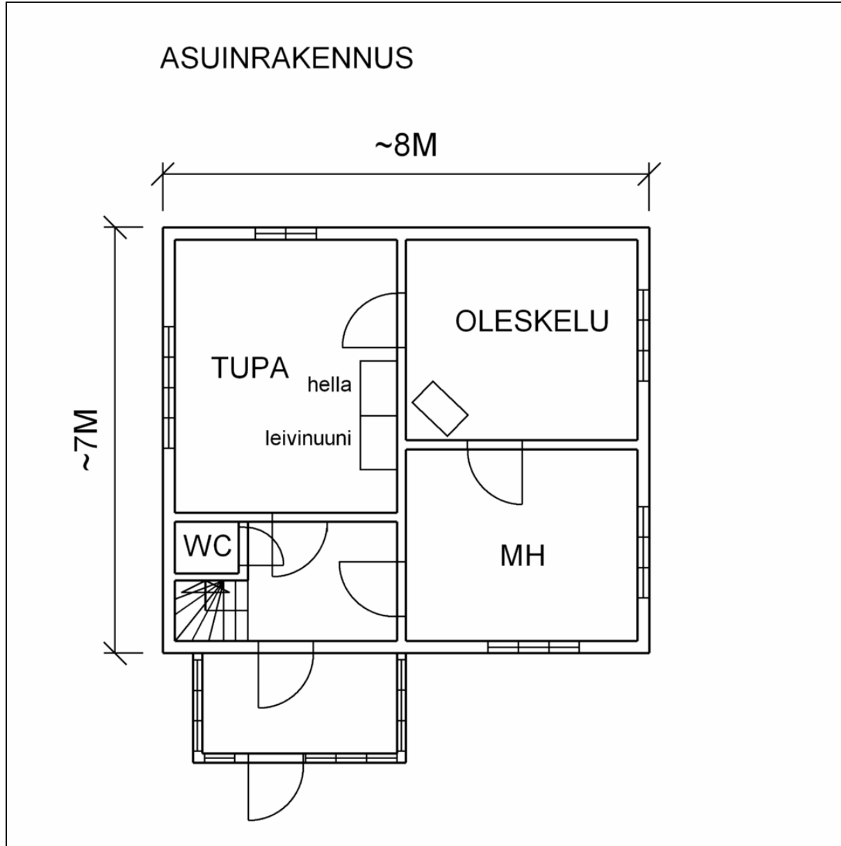
Asuinrakennuksen pohjakaava
