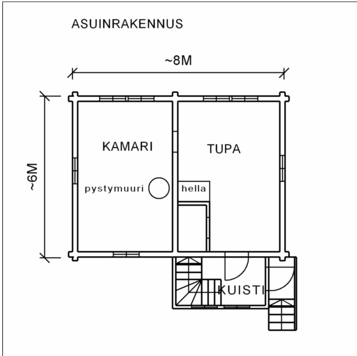
Asuinrakennuksen pohjakaava
