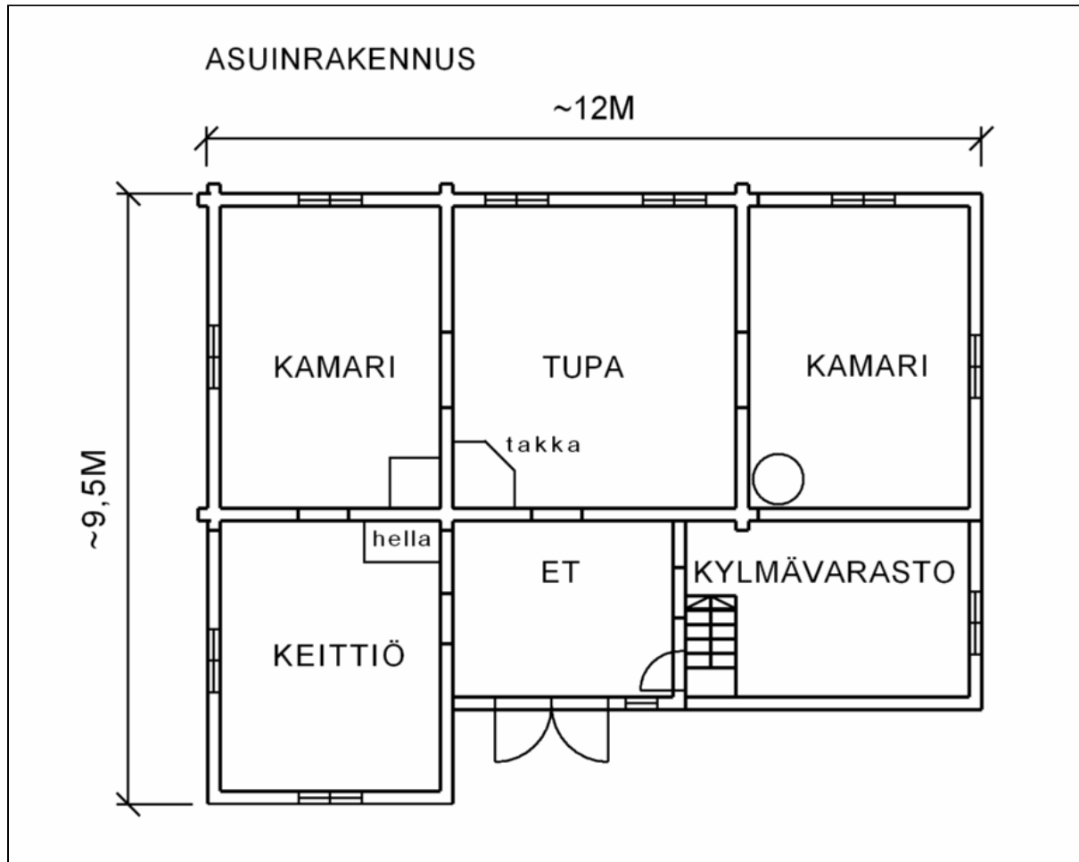
Asuinrakennuksen pohjakaava
