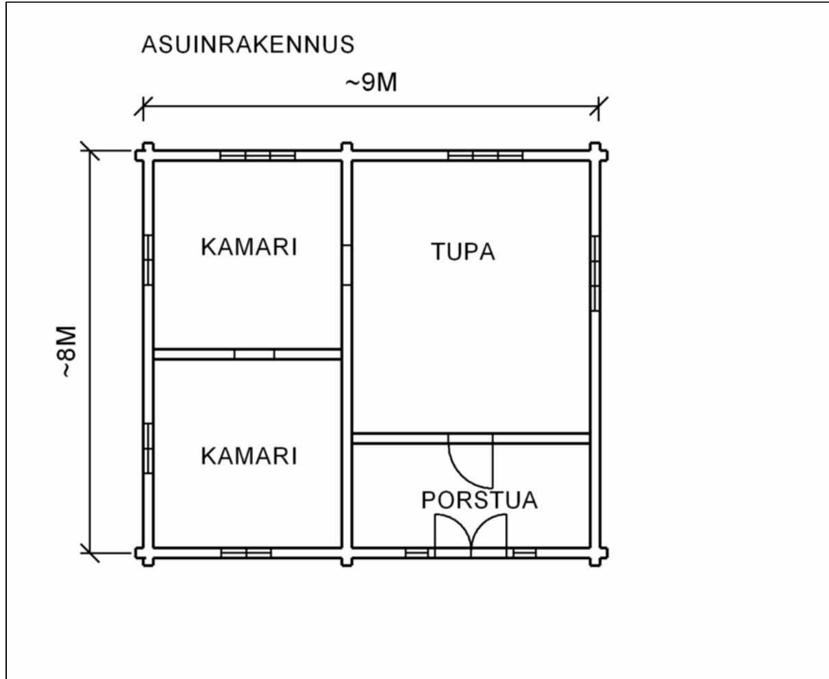
Asuinrakennuksen pohjakaava
