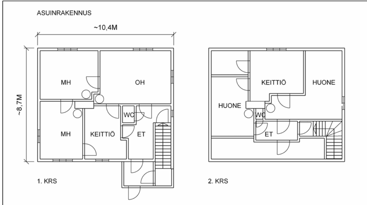
Asuinrakennuksen pohjakaava
