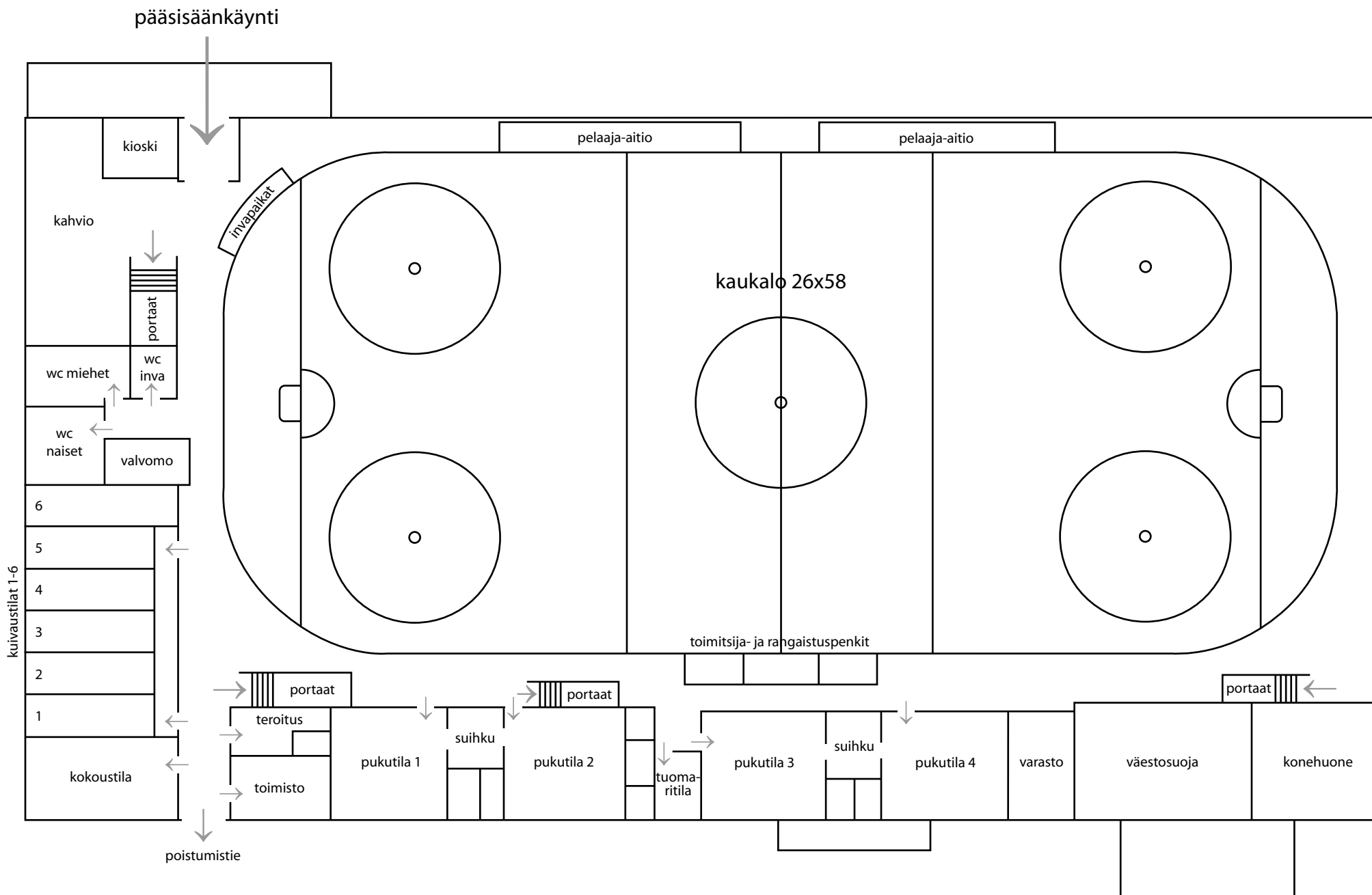
Seinäjoen jäähalli / pohjakerros
